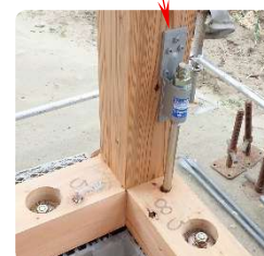
筒型タイプホールダウン金物。15kN用 ビス留め
