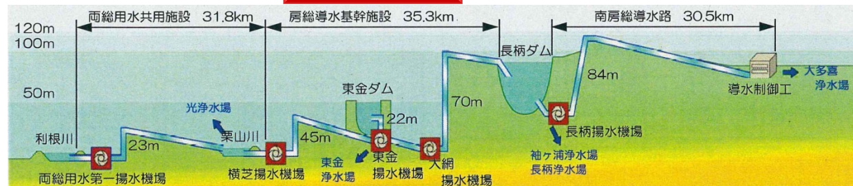
房総導水路断面図 *房総導水路事業パンフレットより。右上地図も同様
