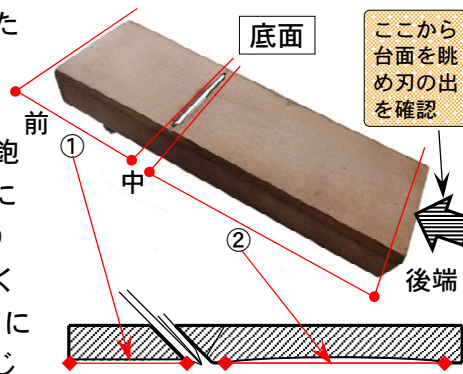
図2 鉋縦断面調整後
