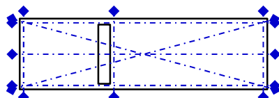
図3 それぞれの青い鎖線方向に差し金等を当て、隙間加減や平らかを確認
